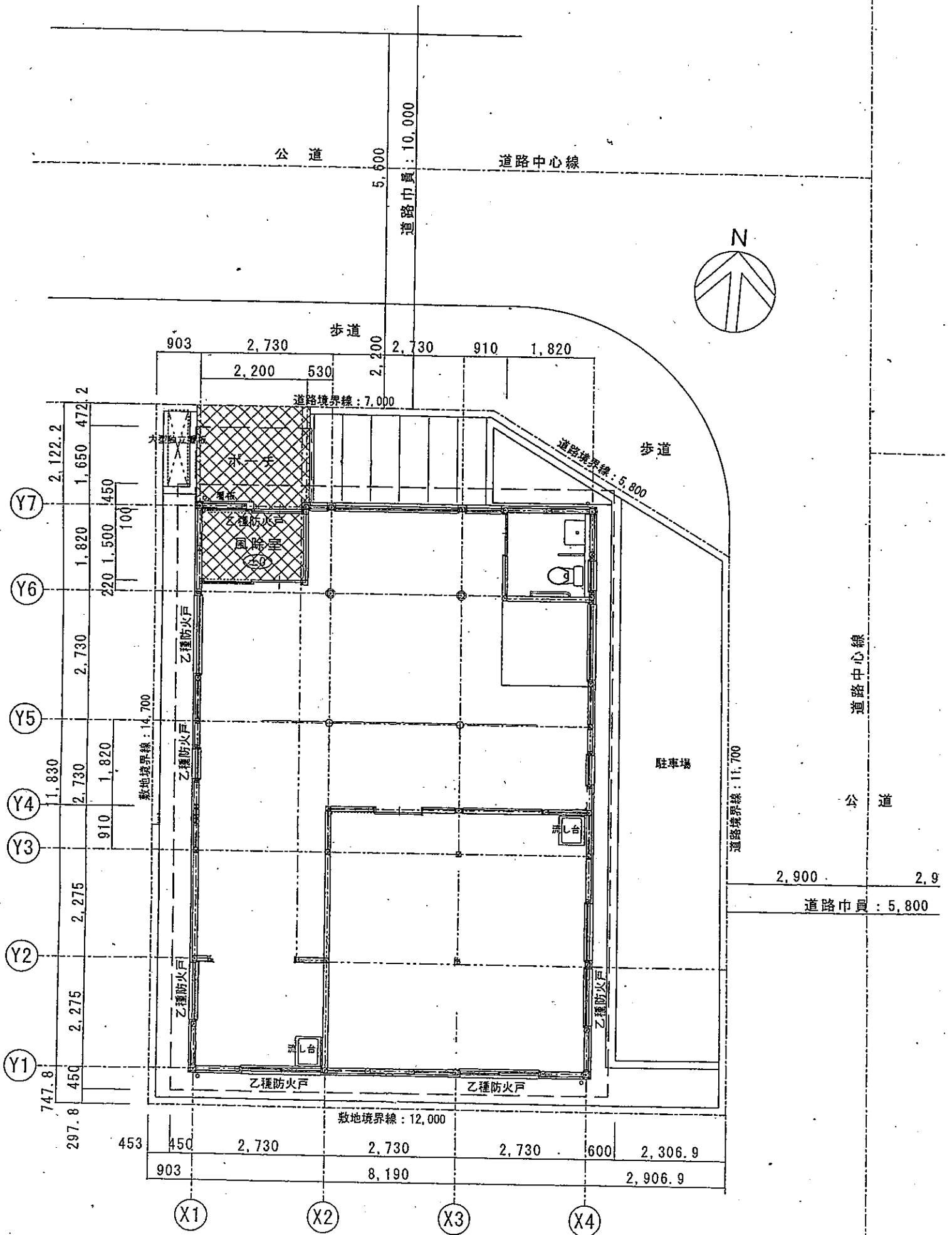
1階平面図 1:100
